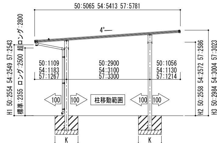
奥行 奥行 寸法図：(単位mm)
